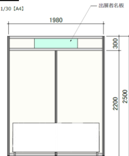
正面図
