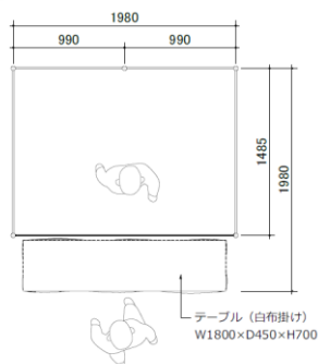
平面図
